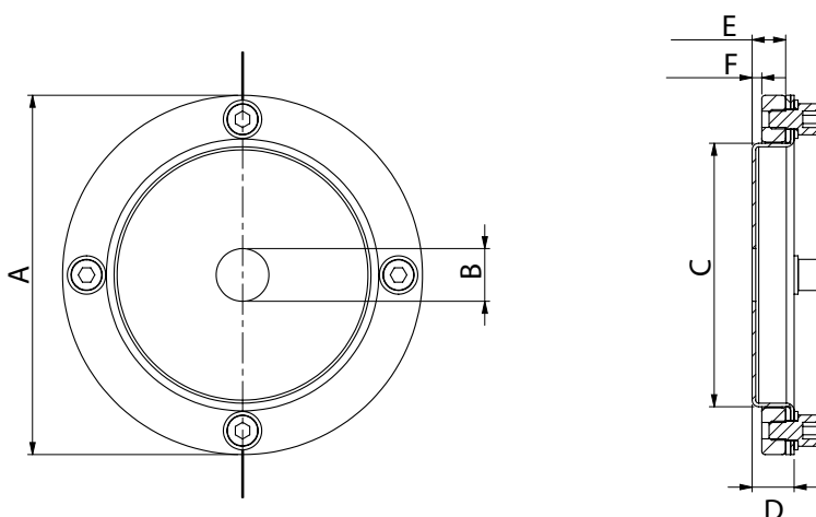
ESPECIFICACIONES DIMENSIONALES
