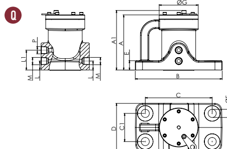
ESPECIFICACIONES DIMENSIONALES
